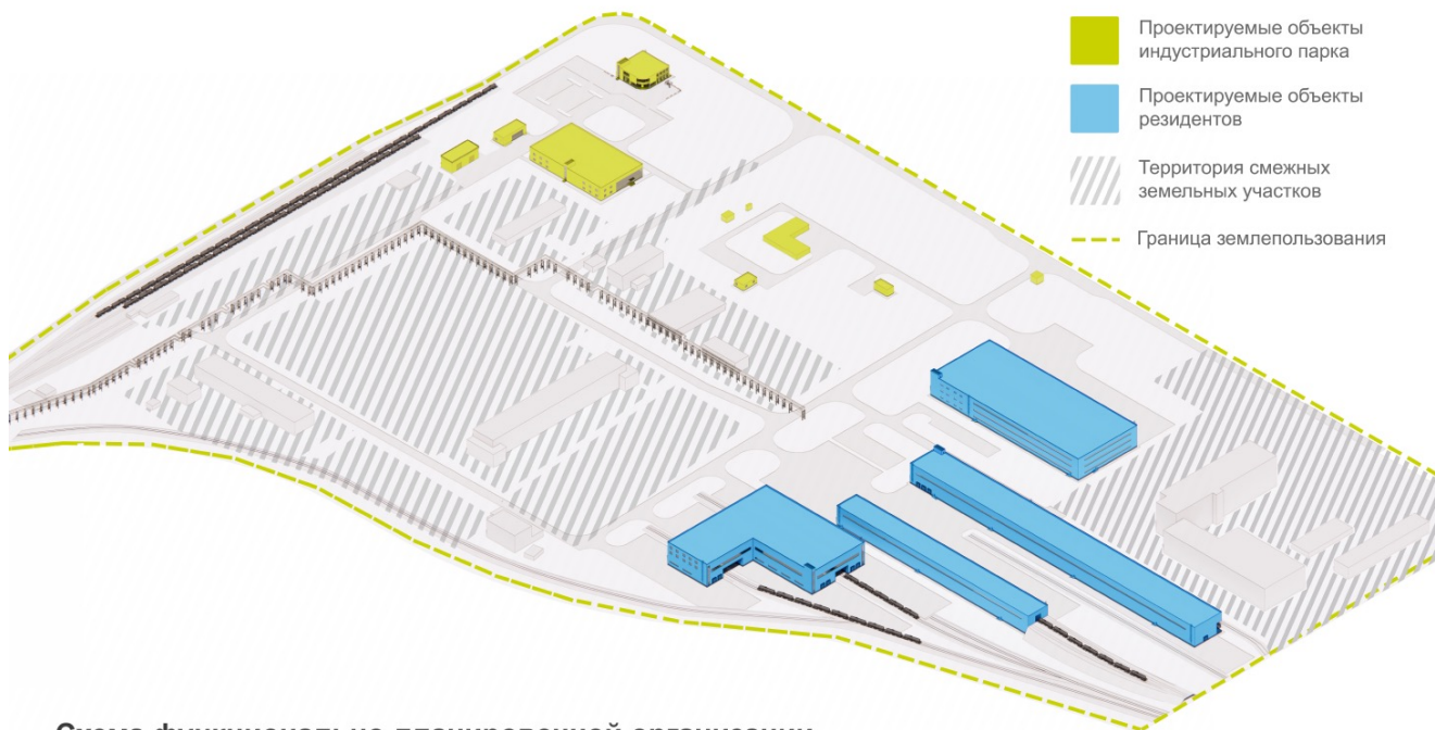
Схема функционально-планировочной организации Территории индустриального парка. Зона резидентов.
